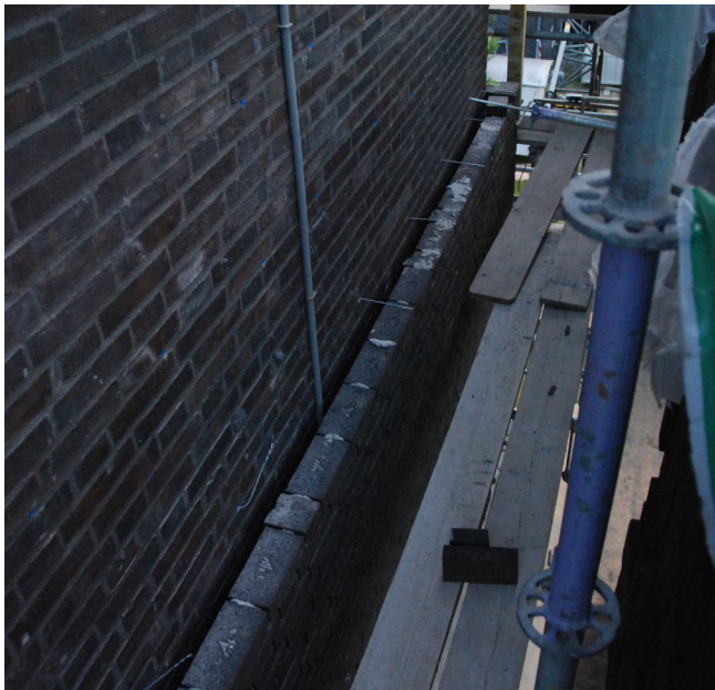
Figuur 3: Gebouw 507. Optrekken van een extra spouw rondom de kopgevel. Construction of extra cavity wall around end façade. Foto: Ruud Kaal
