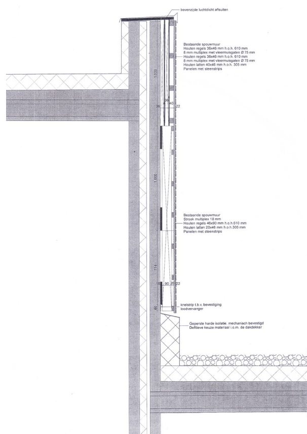
Figuur 5: Opbouw lichte constructie boven plat dak. Composition of light construction over flat roof. Bron: RVB 2013.
