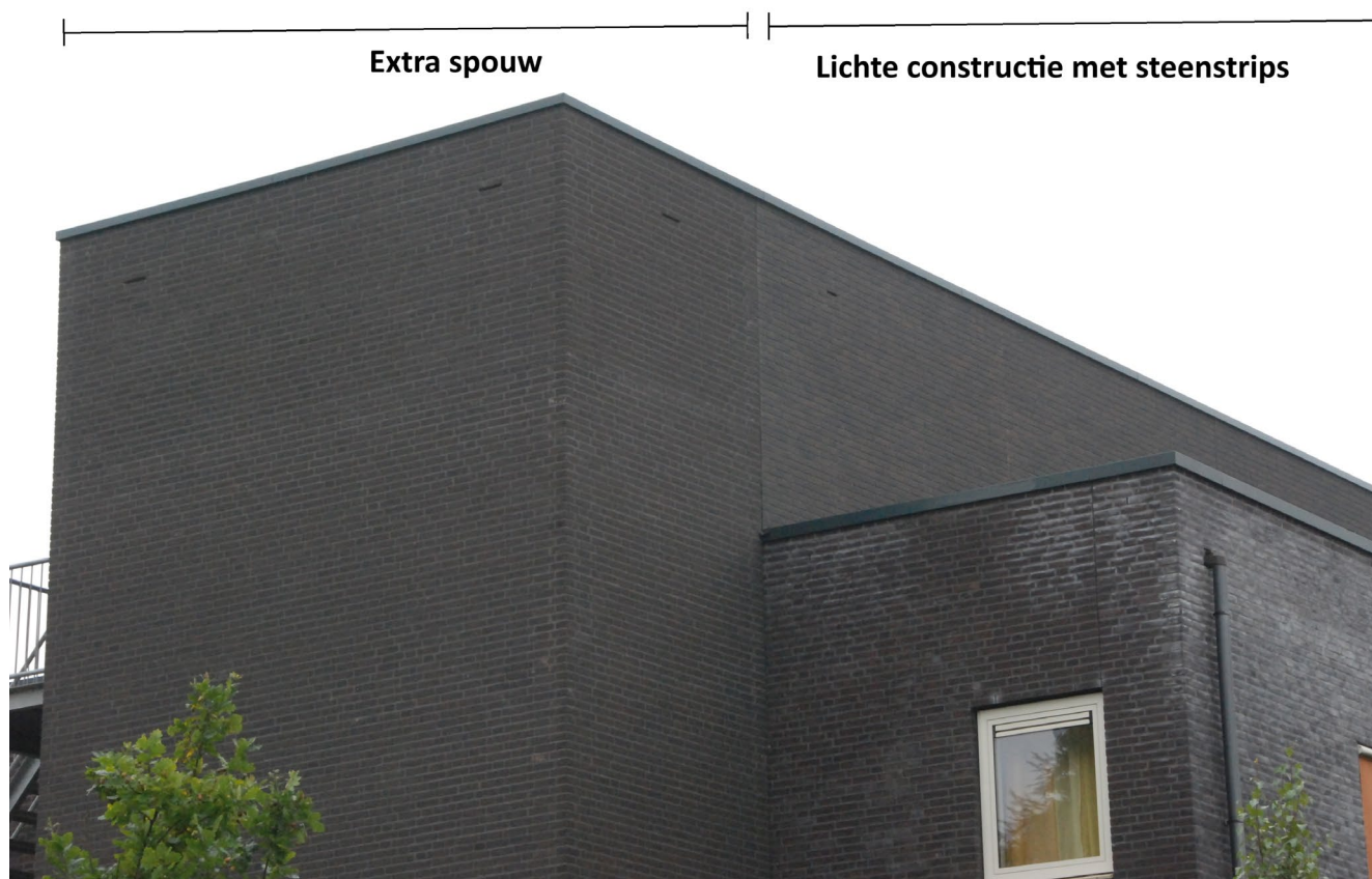
Figuur 2: Gebouw 507. Op en rond de kopgevel is een extra spouw gemetseld met invliegopeningen. Boven het platte dak is deze spouw voortgezet met een lichte constructie van steenstrips op latten met daarin een grote meerlaagse vleermuiskast. Building 507. On and around the end facade, an extra (third) cavity wall has been erected. Over the flat roof, load carrying capacity was insufficient for a cavity wall. Instead, a wall cavity was created with masonry veneer panels over slats and a large multi-layered bat box. Foto: Ruud Kaal
