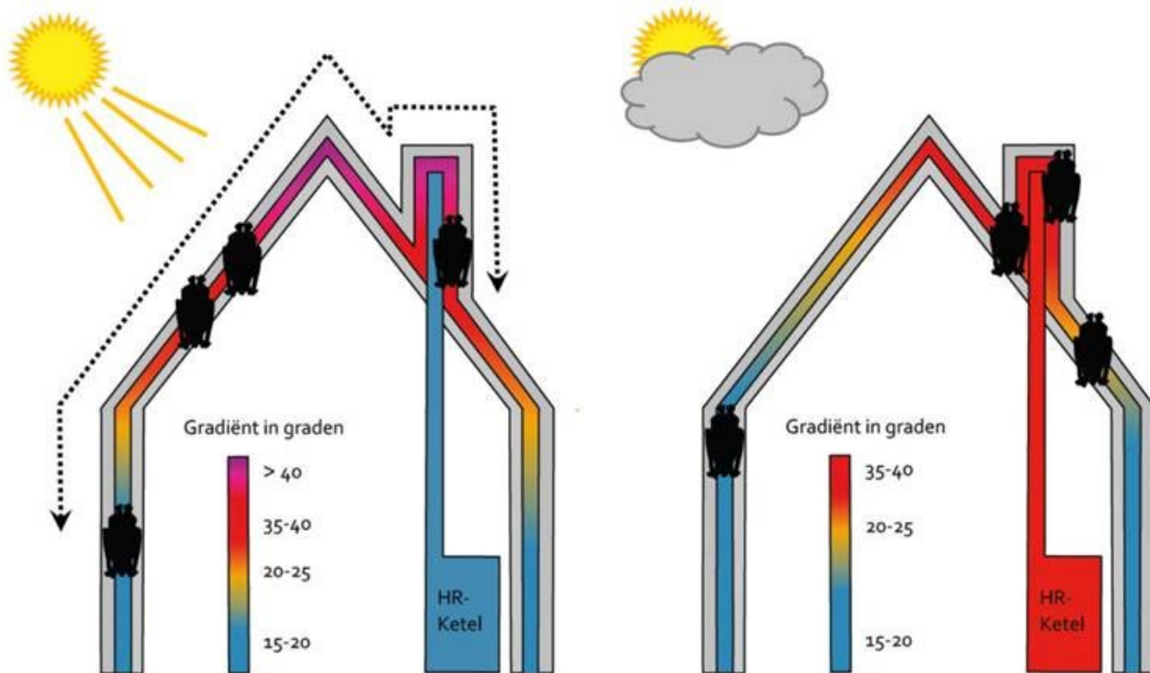
Een slecht geïsoleerd huis uit de jaren '60-'70 biedt veel variatie in microklimaat tijdens zonnige én bewolkte omstandigheden. Uit Haarsma en Janssen (2022).
